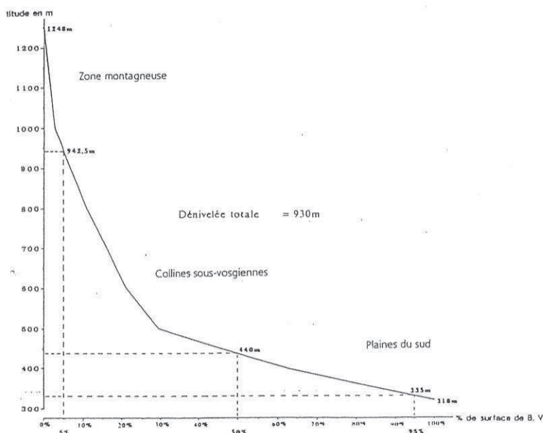
Figure 1: Courbe hypsométrique [4]
